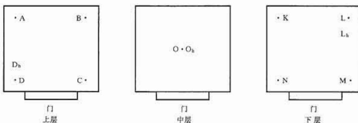
图 1 试验设备容积小于或等于 2\text{ m}^3 时温湿度测量点摆放位置
