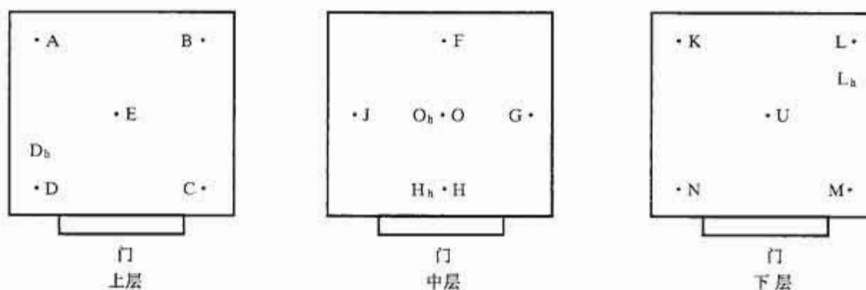
图 2 试验设备容积大于 2\text{ m}^3 时温湿度测量点摆放位置
